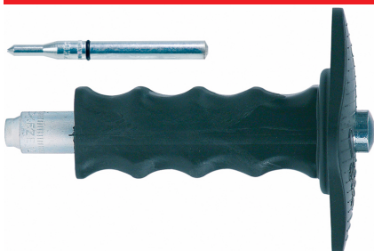
Szerelőszerszám FZE plus
